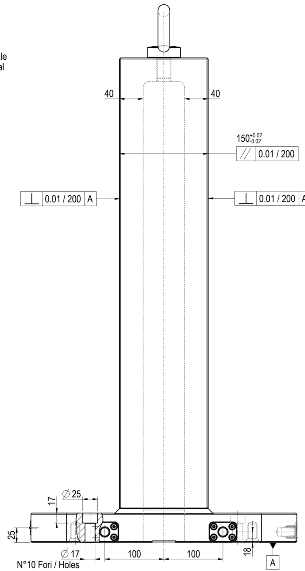
SEZ. B-B
